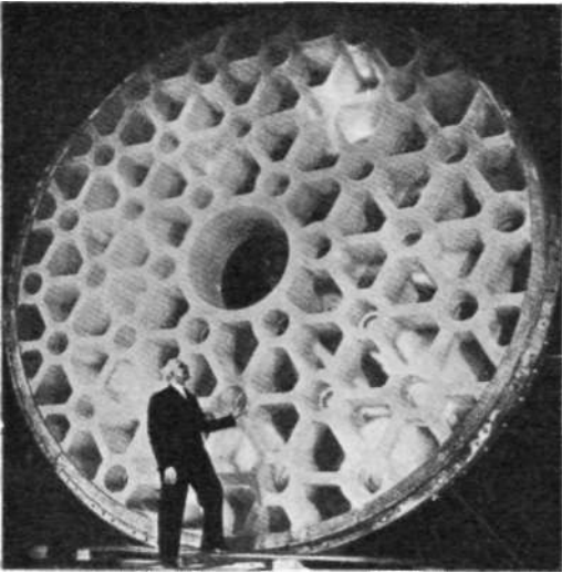
Spejlet til Mt. Palomar-teleskopet, set bagfra. Ribberne giver spejlet øget styrke, medens vægtfølgelsen er relativt ringe.
