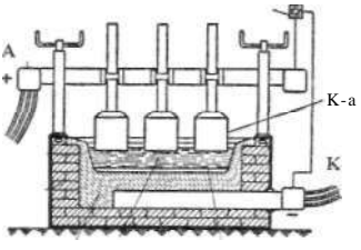
A: anode, K-a: kulanode, K-k: kulkatode. K: kulbund, E: elektrolyt, Fl-a: flydende rå-aluminium. Elektrolytisk udvinning af aluminium.
