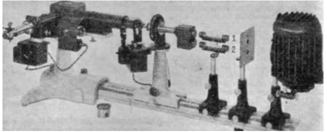
Opstilling til visuel sammenligning af absorptionspektre af lys, der passerer rørene 1 og 2.
