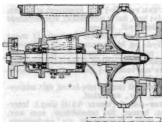
Halvaksial centrifugalpumpe (pumpehjulet på den frie del af akslen).
