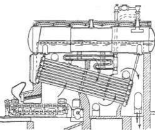
Dampkedel. Babcock & Wilcox-model med skrå vandror.
