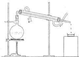
Enkel opstilling til destillation af vand.
