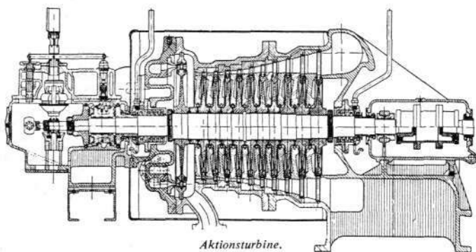
Dampen tilføres gnm. en stuts på turbinehusets underside og strømmer gnm. nogle dyser v. dets venstre ende ud mod løbeskivene på turbineakselens løbehjul, ml. hvilke der i turbinehuset er anbragt skiver m. ledeskive til at rettede dampens bevægelse. Dampafgangen sker v. turbinehusets højre ende.
