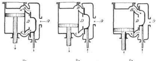
Dampmaskine. Fig. 2.
