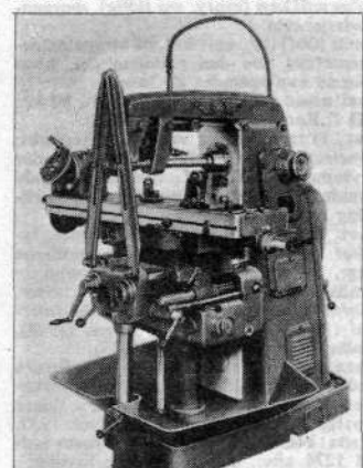
Universalfræsemaskine.
