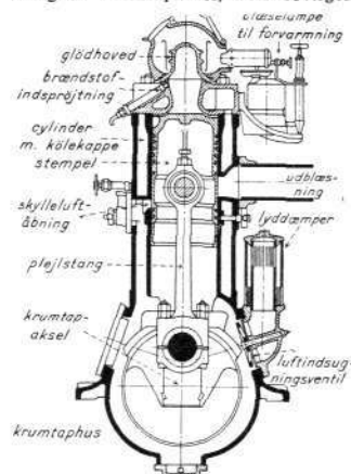
Glødhovedmotor med krumtaphusskyling. Under stemplets opadgående bevægelse indsuges i krumtaphuset luft, der sammentrykkes under stemplets nedadgående bevægelse og, når toppen af stemplet passerer skylleluftåbningen, driver forbrændingsproduktene i cylinderen ud gnm. udblæsningstrøret.
