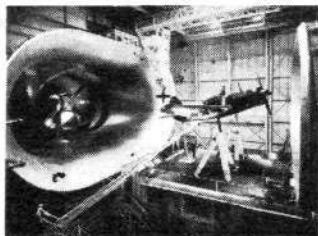
Vindtunnel på flyveteknik forsøgsanstalt.
