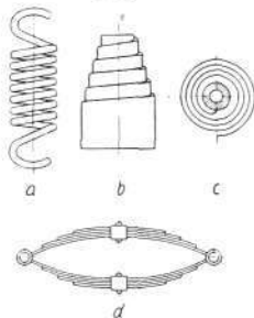
a skruefjeder, b bufferfjeder, c spiral-fjeder, d bladfjeder.
