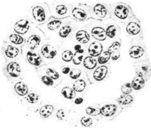
Snit gennem blastula af hvirveldyr.
