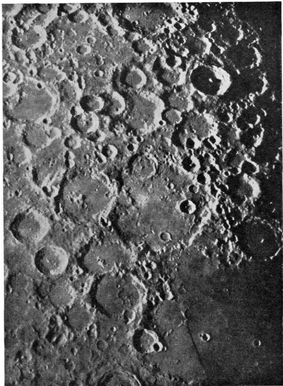
Parti af Månen, efter fotografi af B. Lyot, optaget på observatoriet på Pic du Midi. For oven til højre ses månekrateret Tycho.
