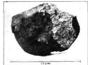
Sten-meteorit, 4 kg, faldet 29. 8. 1878 ved Mern ved Presto. Æneste meteorit fra Danmark. (Mineralogisk Museum, Kbh.)
