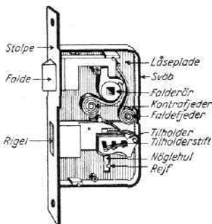
Indstikken lås med 4 tilholdere af Chubb-systemet.
