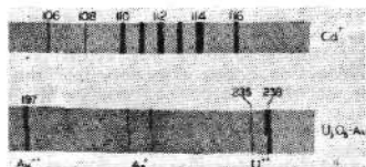
Massespektrum af isotoperne af cadmium (øverst) og uran (nederst).
