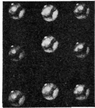
Planeten Mars. Optagelser taget med korte mellemrum for at udnytte de kortvarige perioder med rolig luft, der giver de bedste billeder.
