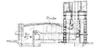
Herdovn. Smelteovn. Flammen slår over broen forbi ovndøren og stryger langs herden. Det smeltede metal aftappes t. h.
