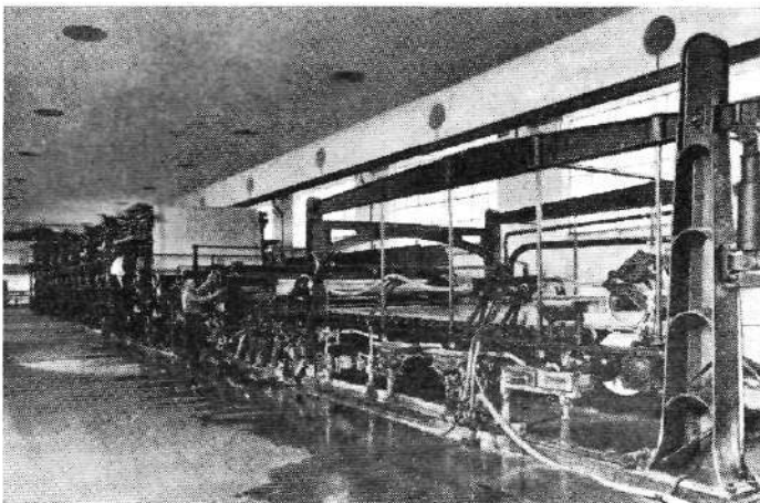
Papirmaskine.
