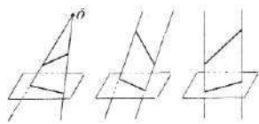
Central-, parallel- og retvinklet projektion.
