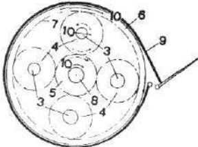
Skitse af planetgear, fig. 1 sidebillede, fig. 2 lodret billede. - 1 drivaksel med fastkilet svinghjul 2, hvori der er fastgjort tappe 3. På tappene sidder planet-hjulene 4, der er i indgribning med solhjulet 5 og tandkransen 7 på kapslen 6, som kan fastholdes med bremsebåndet 9. 8 er den drejende aksel, hvorpå solhjulet 5 er fastkilet. Når bremsebåndet er løst, vil delene drejes som vist med pile 10, men følge de punkterede linier, når bremsebåndet er trukket an.
