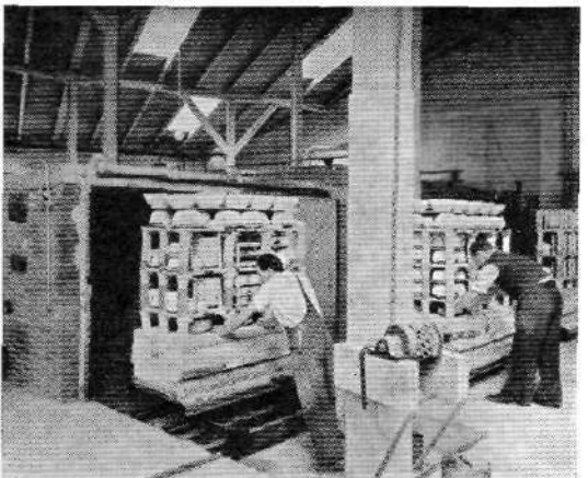
Tunnelovn for fajance.
