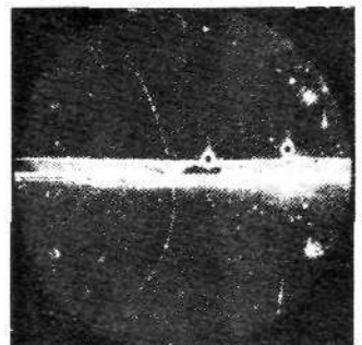
Tagekammerfoto af positron, der passerer en blyplade og krummes af et magnetfelt.
