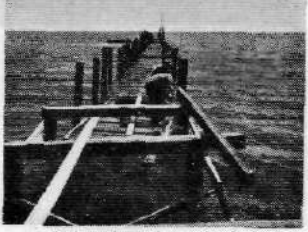
Pæleværk under opførelse.
