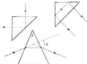
Prisme(fys.); nederst: brydning ip; øverst: totalreflektion i p (enkelt og dobbelt).
