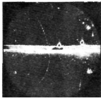
Tage kammer foto a/positron, der passerer en bly plade og krummes af et magnetfelt.
