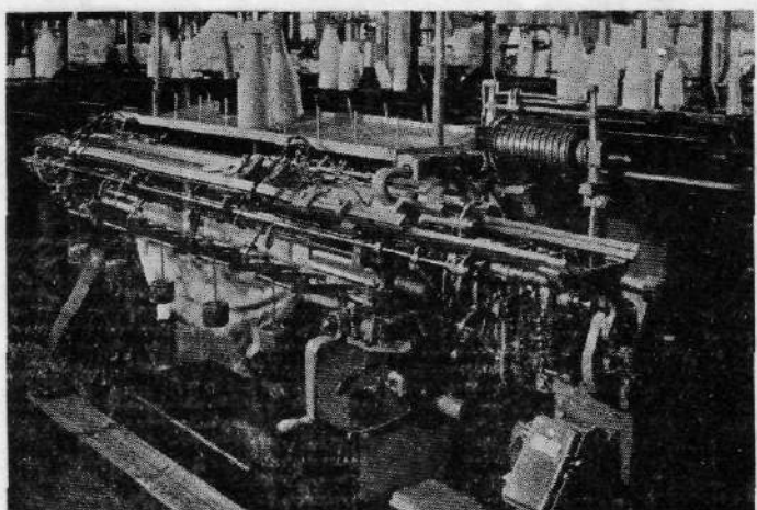
Helautomatisk fladstrikkemaskine med dobbelt system til fremstilling af trikotage. Da alle omskiftninger sker automatisk, kan en arbejder betjene fl. maskiner ad gangen.
