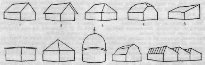
1 alm. sædetag, 2 sædetag med udnæns, 3 valmtag, 4 halvvalmtag, 5 halvtog, 6 fladt tag, 7 pyramidetag el. telttag, 8 kuppeltag, 9 mansardtag, 10 shedtag.
