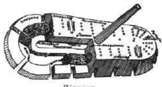
Ringovn.
