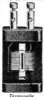
Termosøjle.
