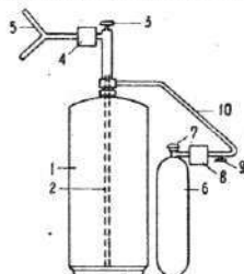
Tågesyrebeholder. 1. beholder, 2. stigerør, 3. stopventil m. filter, 4. fjernbetjeningsventil, 5. gaffelrør m. forstøvningsdyser, 6. tryklufflaske, 7. stopventil, 8. reduktionsventil og trykmåler, 9. afspæringsventil, 10. armeret slange.
