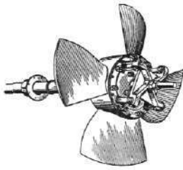
Turbine med indstilleligt skovlhjul.
