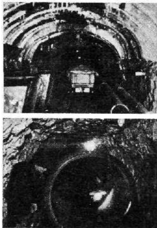
Kloaktunnel, Øresund. Øverst: del af betonret vesttunnel. Nederst: rørlægning.
