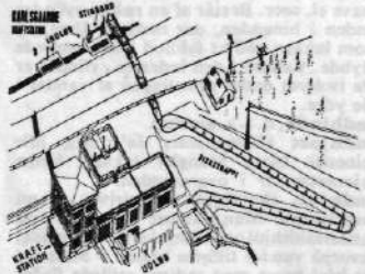
Karlsgårde vandkraftanlæg ved Holme Å øst for Varde.
