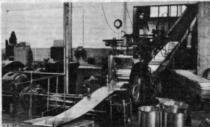
Koldvalsnings af aluminiumbånd.
