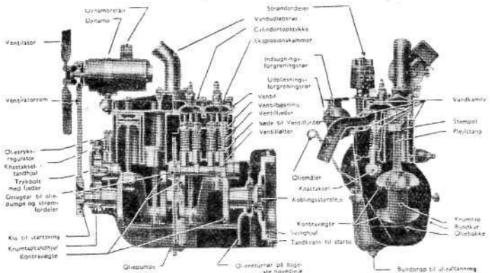
Længde- og tværsnit af 4-cylinders 21 HK Ford motor
