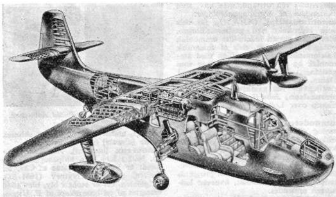
Amfibieflyvemaskine, Short Sealand (England).
