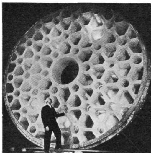
Spejlet til Mt. Palomar-teleskopet, set bagfra. Ribberne giver spejlet øget styrke, medens vægtførelsen er relativt ringe.
