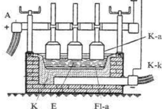
A: anode, K-a: kulanode, K-k: kulkatode, K: kulbund, E: elektrolyt, Fl-a: flydende rå-aluminium.
