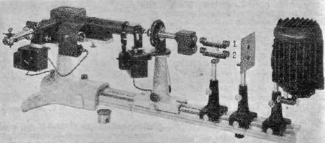
Opstilling til visuel sammenligning af absorptionspektre af lys, der passerer rorene 1 og 2.
