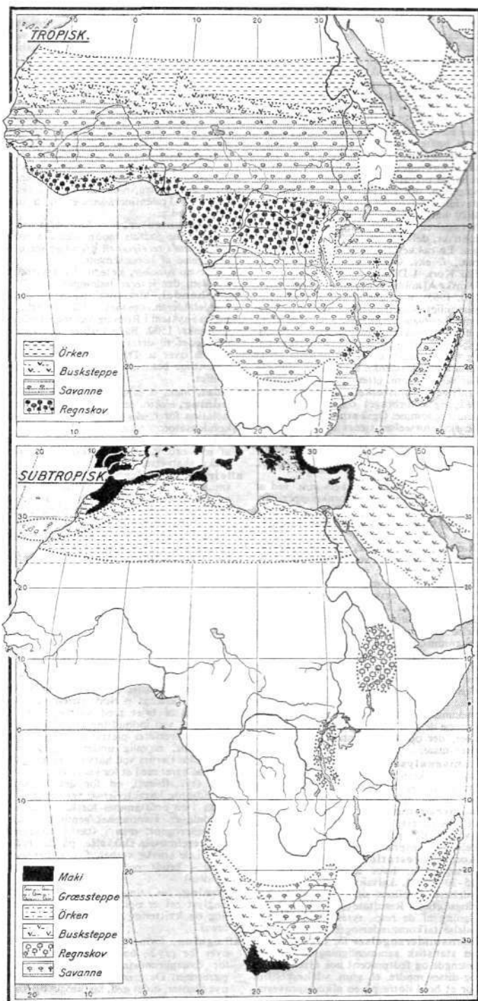
Maalestok 1:80 000 000 Udarbejdsle: J. Humlum Afrika: plantegeografiske regioner. (Efter M. Vahl)
