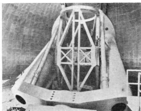
Spejlteleskopet på Mt. Palomar, det største eksisterende. Hovedspejlets diameter er 5 meter.
