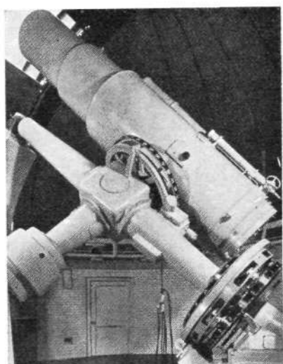
Schmidt-teleskopet på Warner and Swasey Observatoriet i Cleveland, særlig egnet til fot. af store arealer af himlen.
