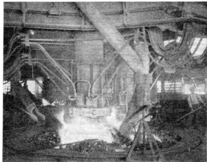
Trefaset elektrisk smelteovn til fremstilling af aluminiumoksyd.
