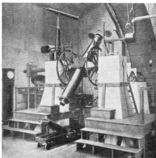
Washington Observatoriets meridiankreds, benyttes til bestemmelser af himmellegemers positioner.
