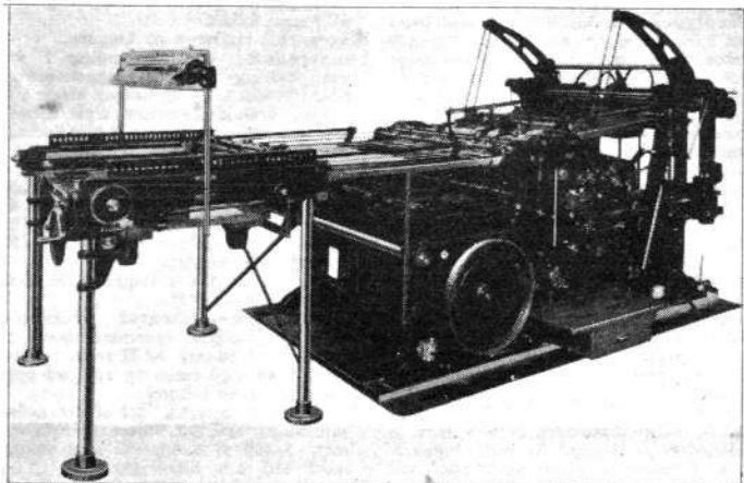
Moderne hurtiggående bogtrykpresser med selvpålegningsapparat. Kørehastighed 1-3000 tryk i timen.
