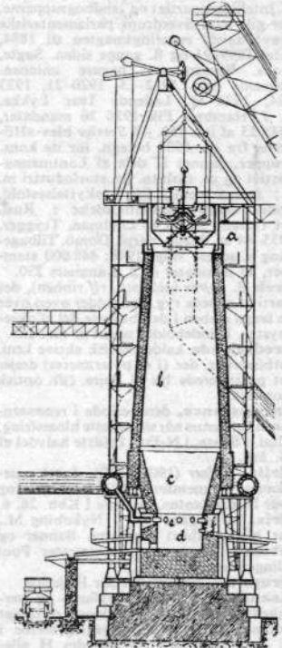
Snit gennem højovn.
