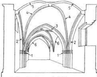
1. Kragbånd 4. Ribbe 2. Skjoldbue 5. Hvalvkappe 3. Gjortbue 6. Fødselslinie
