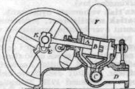
A cylinder, B stempel, C og D til- og afgangsrør, K krumtap, E aksel, F vindkedel til dæmpning af vandstød.
