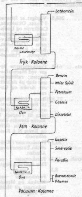
Skematisk fremstilling af moderne kontinuerligt destillationsanlæg (pipe-still) for jordolie. (Laboratoriet for Almen Teknisk Kemi, Polyteknisk Læreanstalt).
