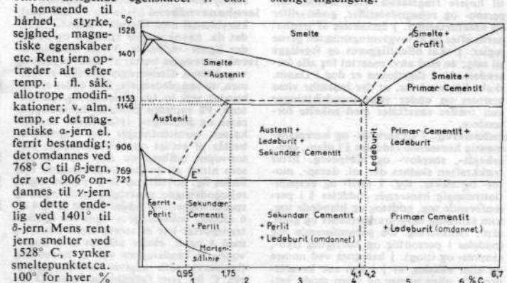
Jernkulfstøfdiagram med angivelse af strukturbestanddelene, kulstofprocenten og de forsk. overgangstemp. E og E' er henholdsvis eutektisk og eutektoidt punkt. Den stiplede linie angiver forholdene ved meget langsom afkøling (grafitdannelse).
