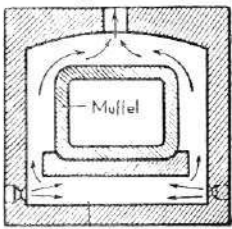
Forbrændingsrum Åbnindelig muffelovn.
