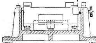
Fræsekasse.
