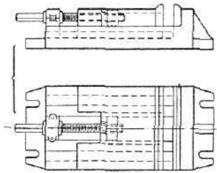
Maskinskruestik.
