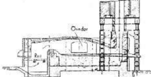
Herdovn. Smelteovn. Flammen slår over herden forbi ovdøren og stryger langs herden. De smeltede metal aftappes t. h.
