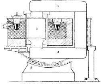
Elektroovn. Induktionsovn. a transformatorkerne, b primærvinding, c ringformet smeltende, d kippemekanisme.
